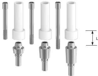
Stég fej, külső kúpos, átmenő csavarral
